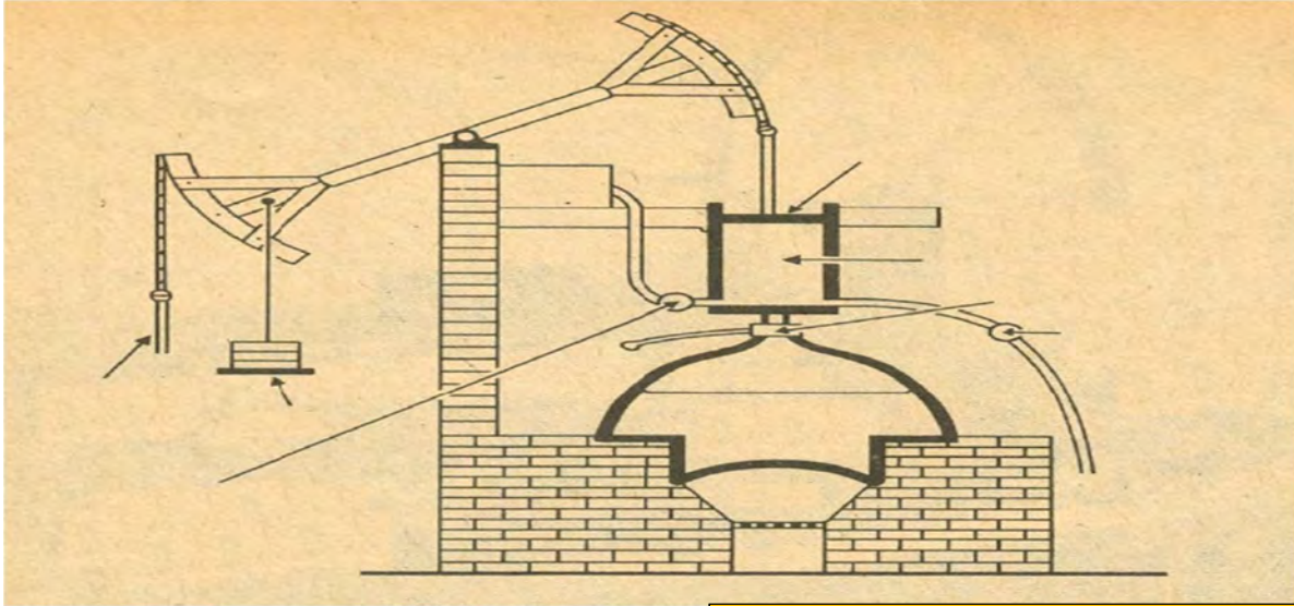
پۆمپى ھەلئى نېوكومن بە ھۆى جولەى دەوهرىى ياخود جولەى يەك لەدواى يەك
